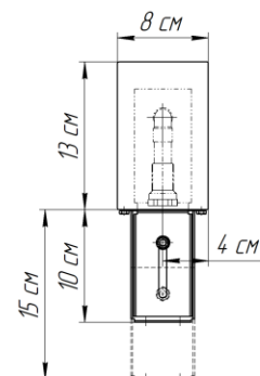
Исполнение "рв" (регулируемая высота)
