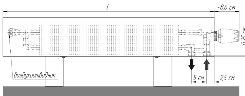
Вид для исполнения "нв" (нерегулируемая высота)
