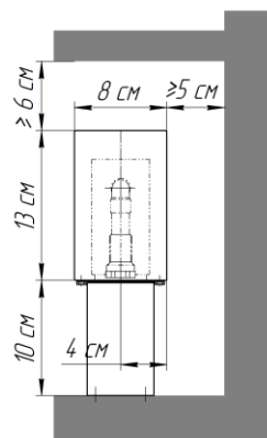
Исполнение "нв" (нерегулируемая высота)
