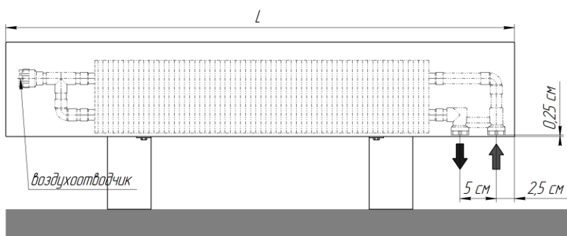
Вид для исполнения "нв" (нерегулируемая высота)
